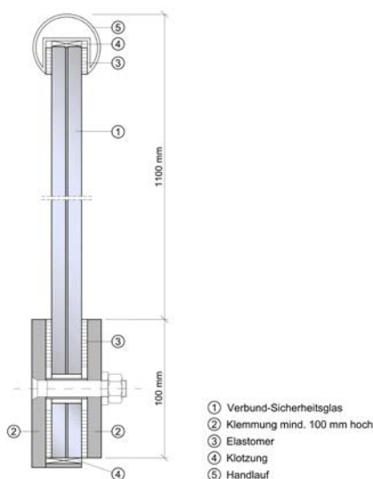
Abbildung 1: eingespannte Verglasung mit Handlauf
