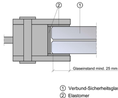
Abbildung 5: Querschnitt Randklemmhalter
