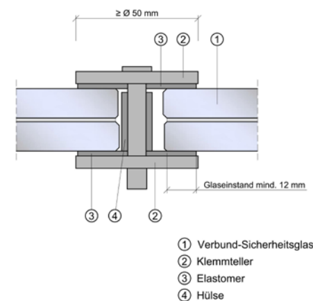
Abbildung 4: Querschnitt Tellerhalter
